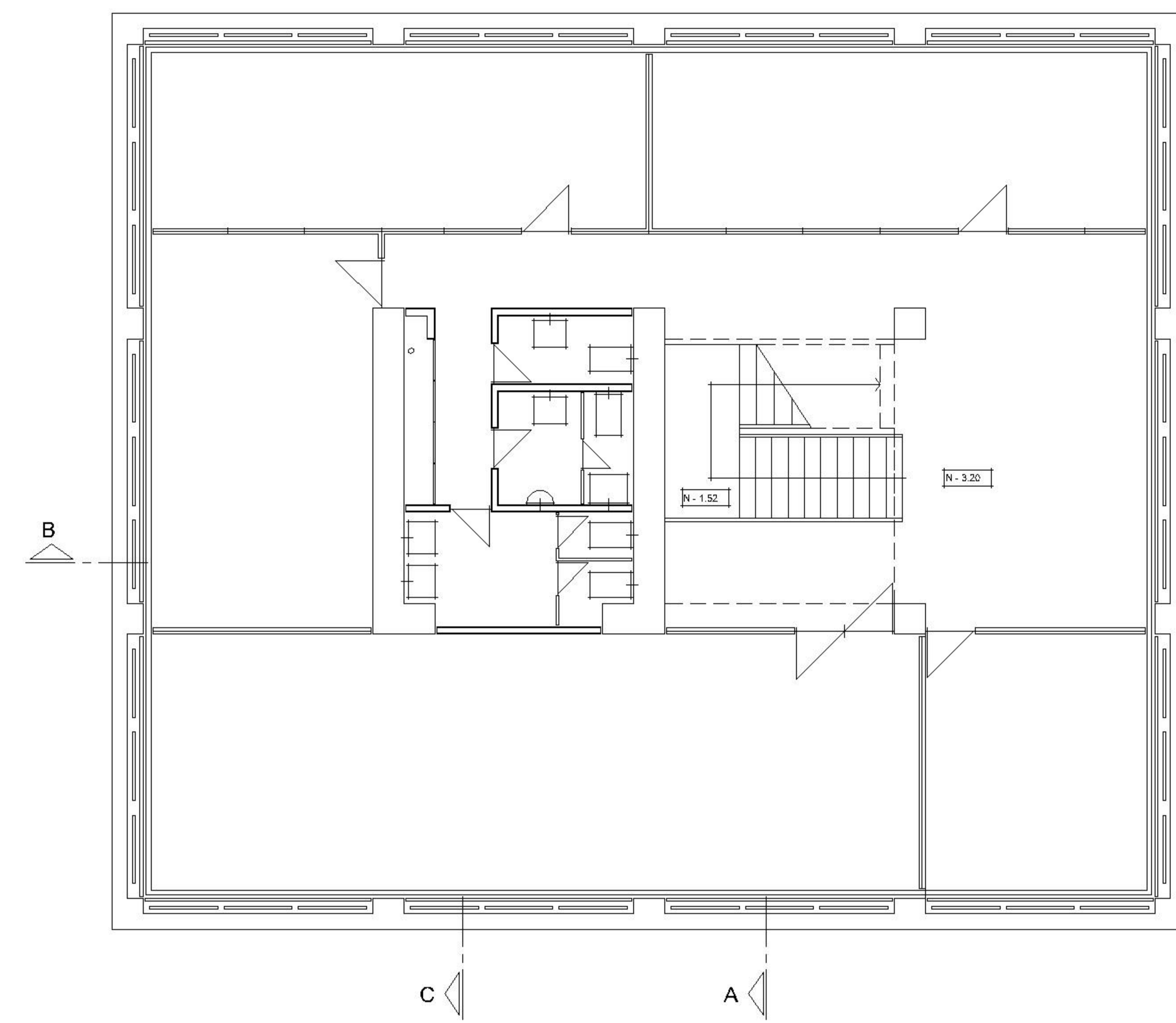
PLANTA NIVEL -1 N -3.20 ESCALA 1 : 200
