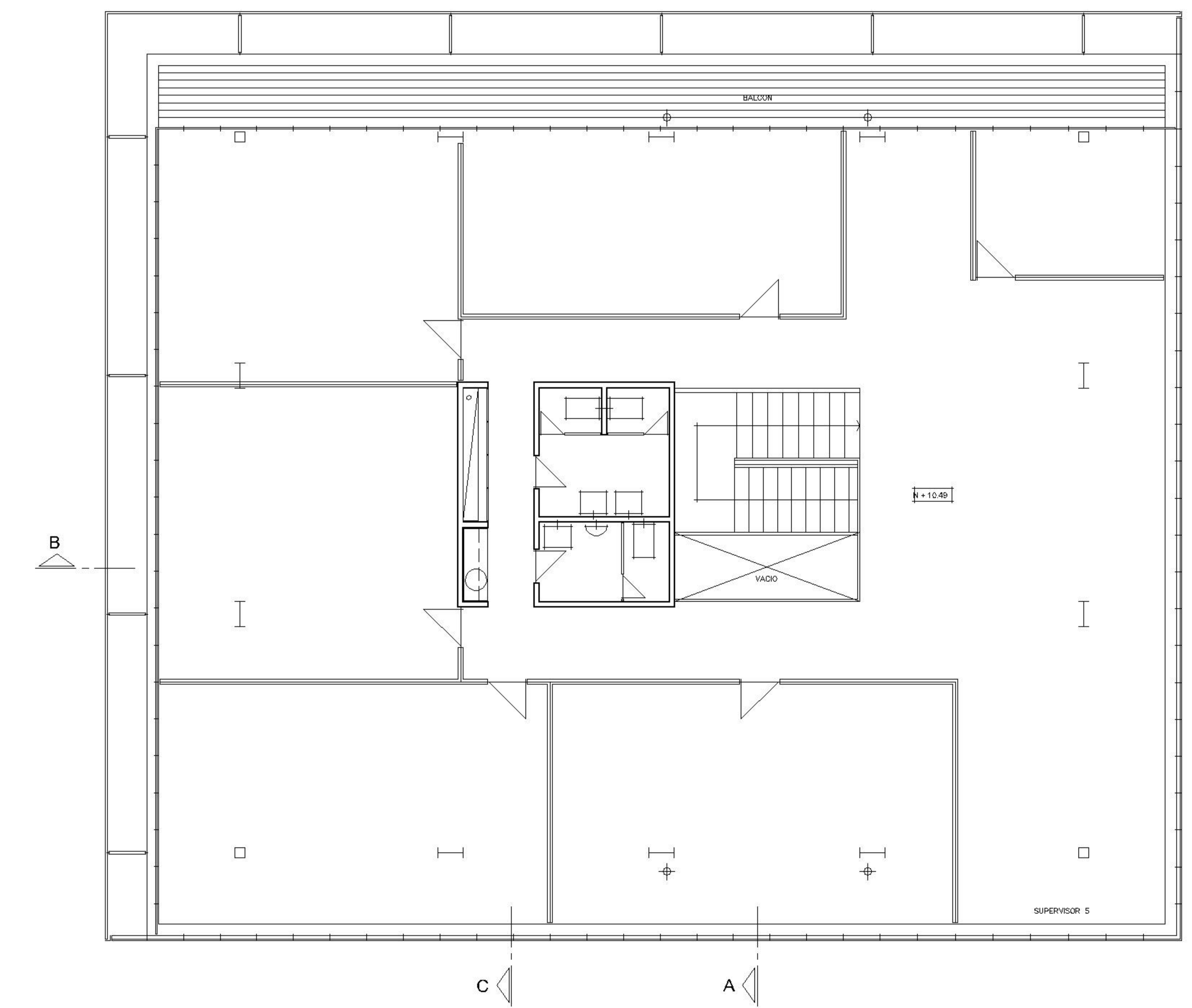
PLANTA NIVEL +5 N +10.49 ESCALA 1 : 200
