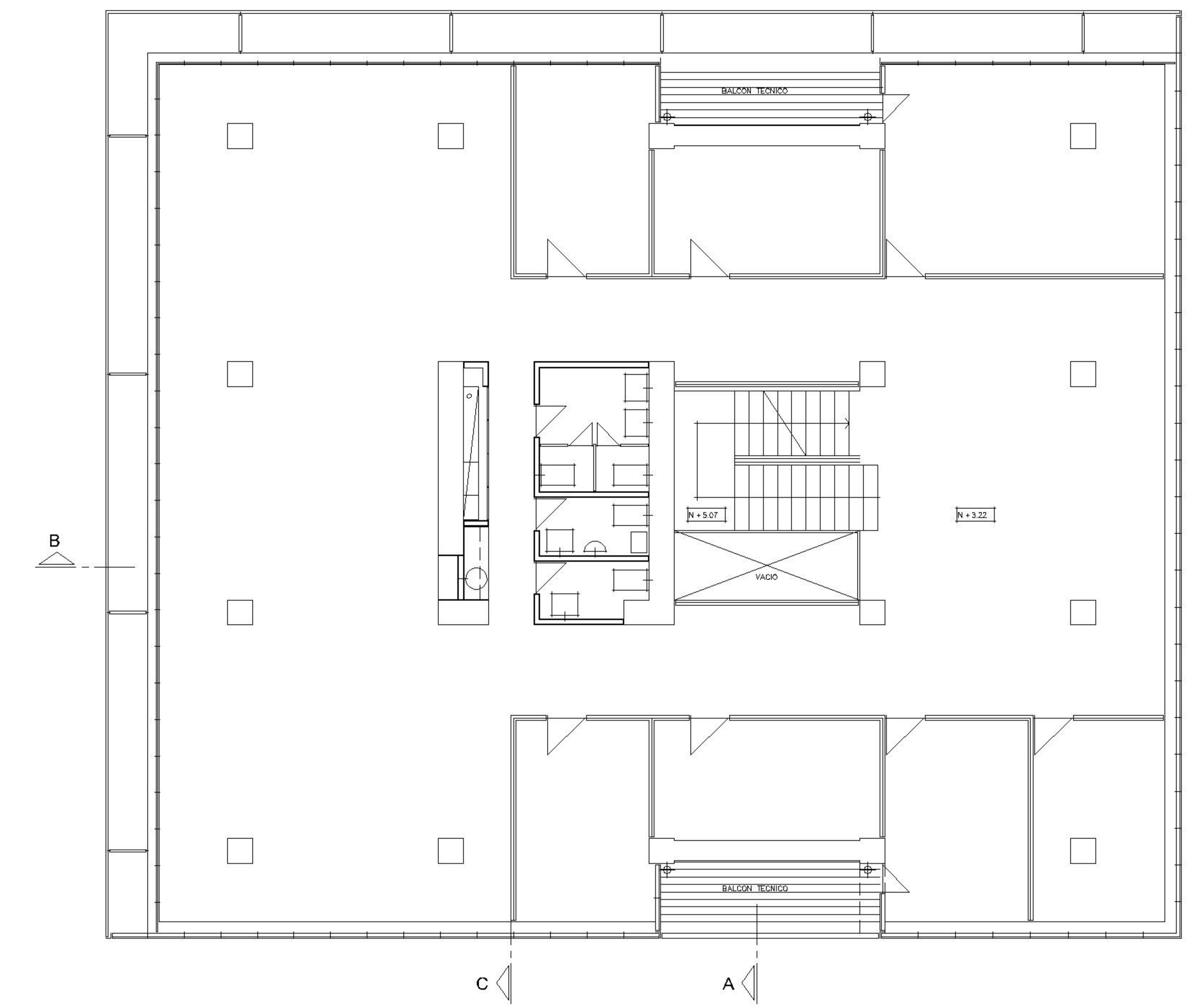
PLANTA NIVEL +3 N +3.22 ESCALA 1 : 200
