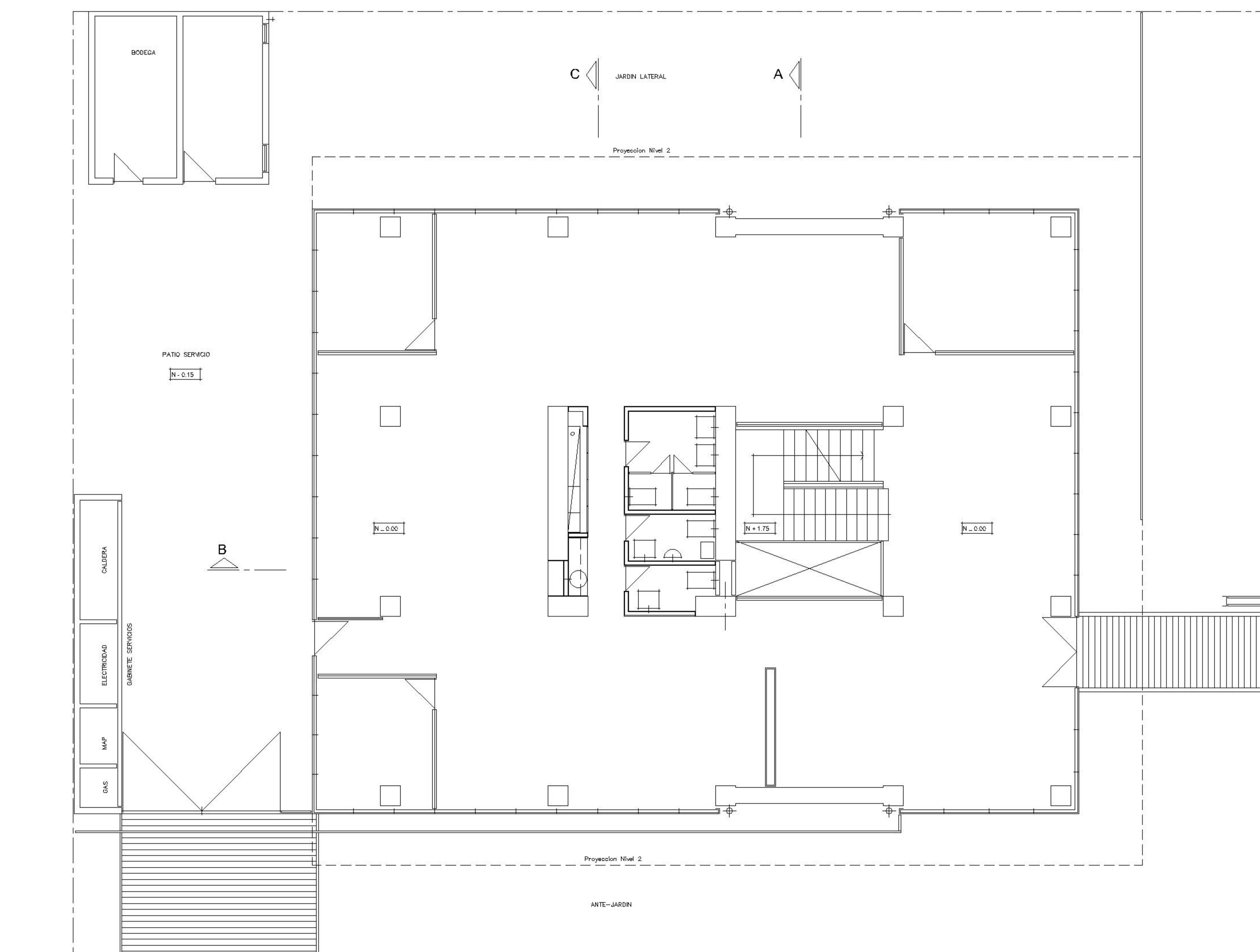
PLANTA NIVEL -1 N -3.20 ESCALA 1 : 200
