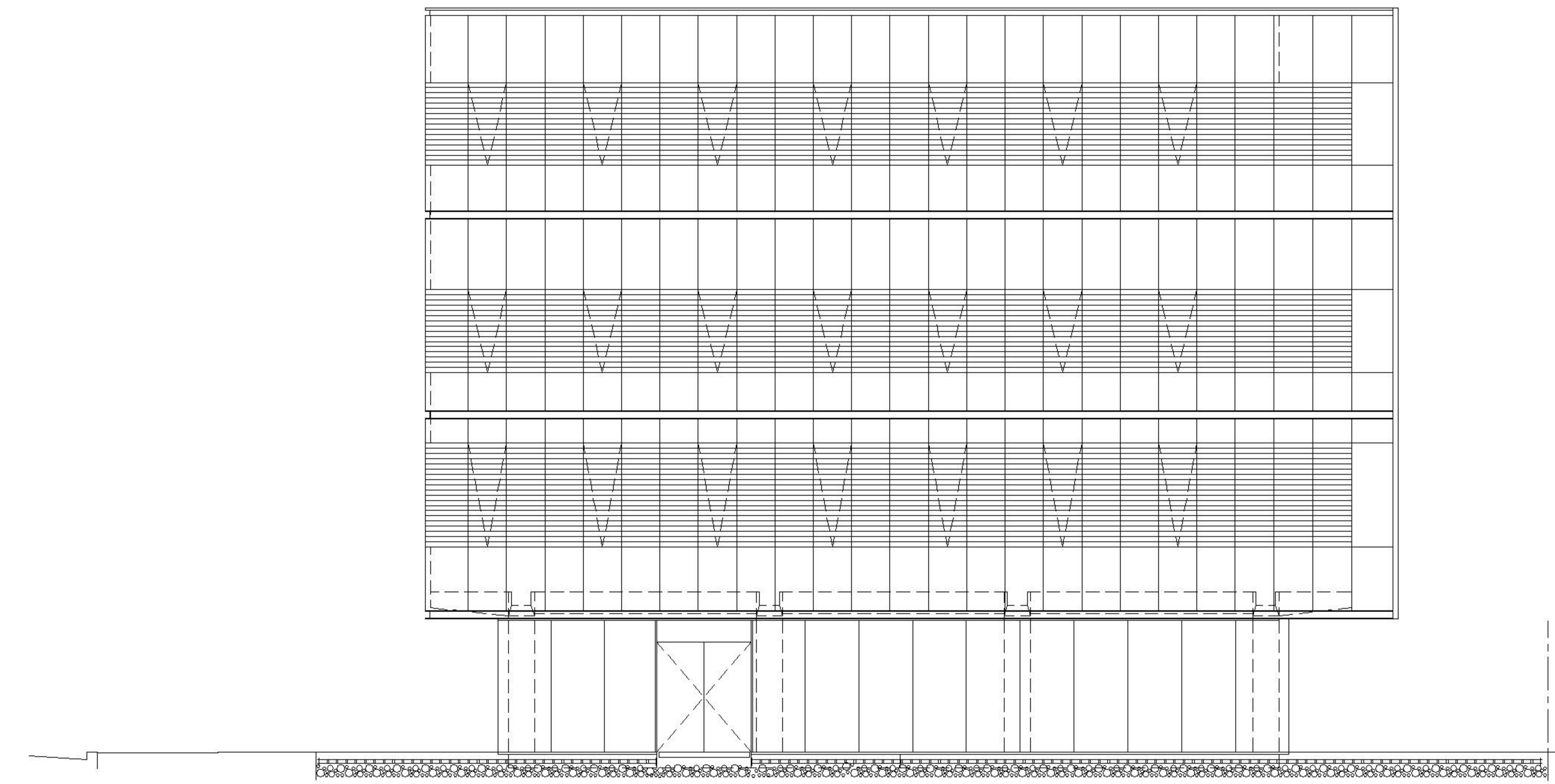
ELEVACIÓN ORIENTE
