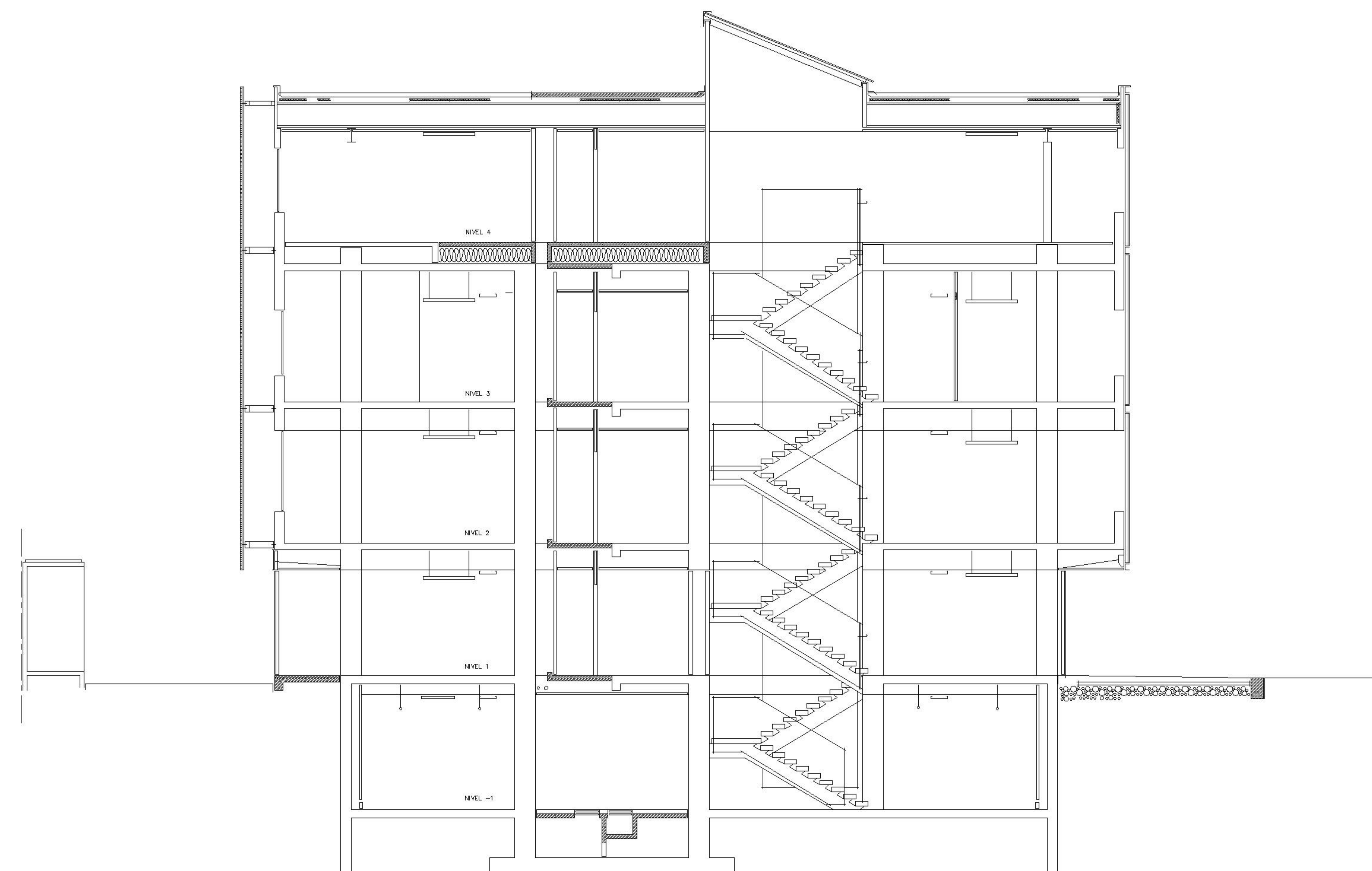
CORTE B - B
